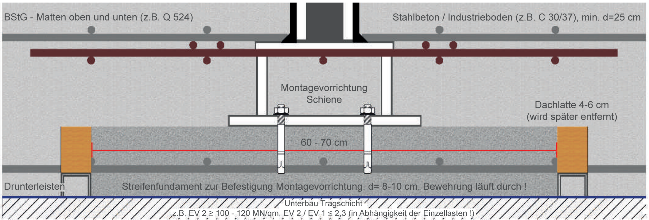
Schiene auf Halterung
