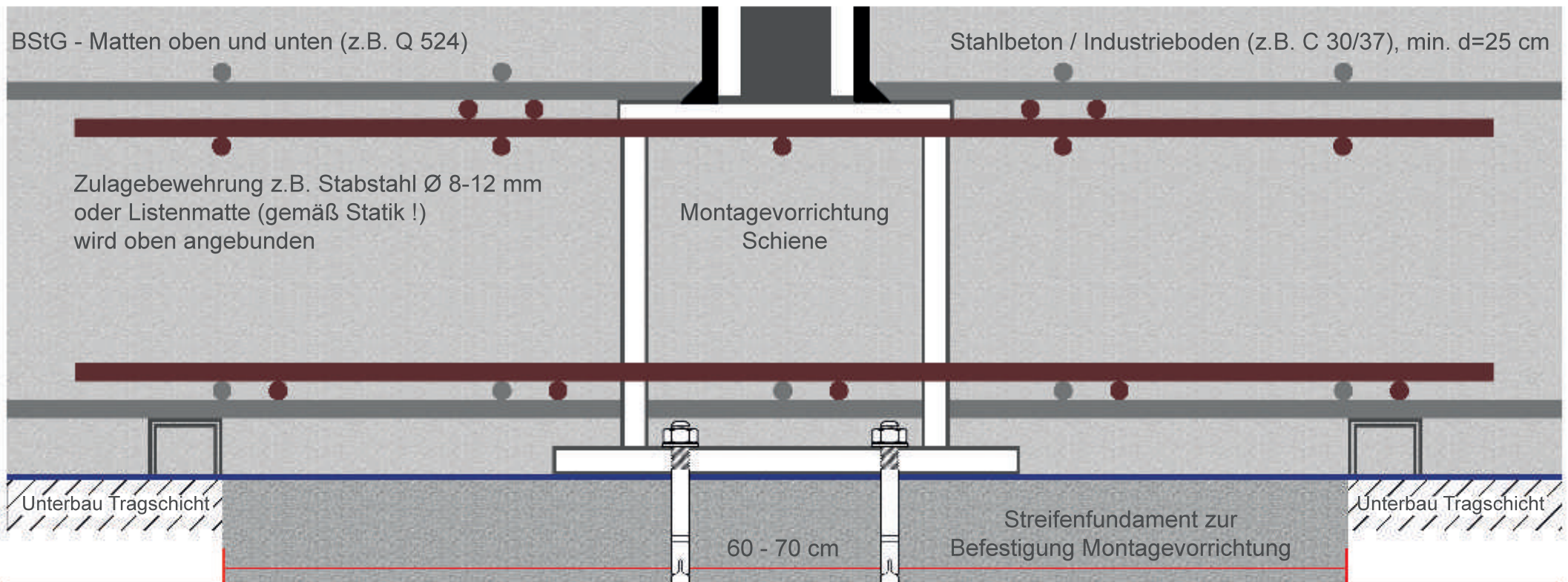
Schiene auf Halterung
